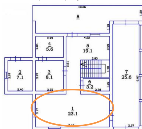
Позтажный план
