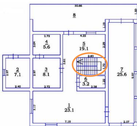
Поэтажный план
