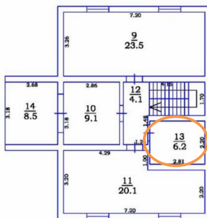
Позэтажны план
