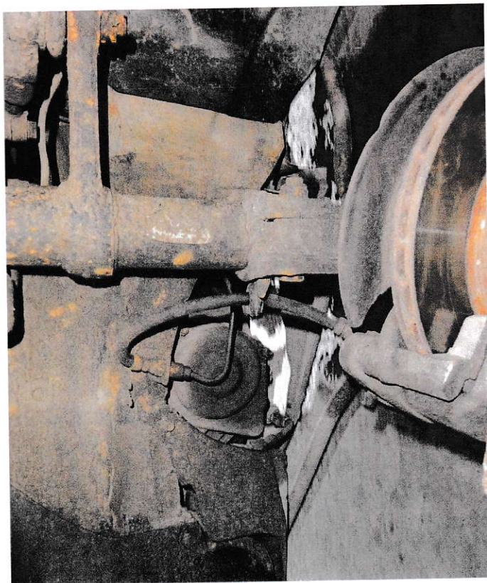
Левая часть передней подвески.
